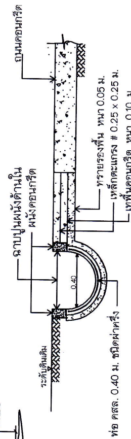
รูปตัดร่องระบายน้ำ NO SCALE
